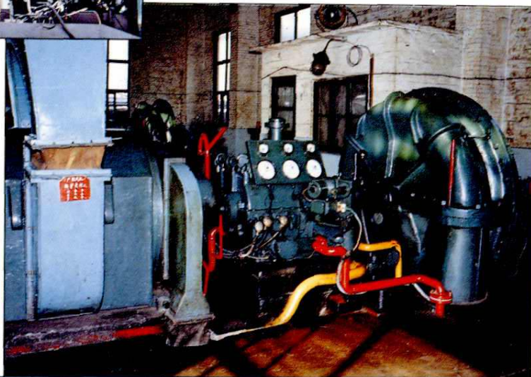
液力耦合器
