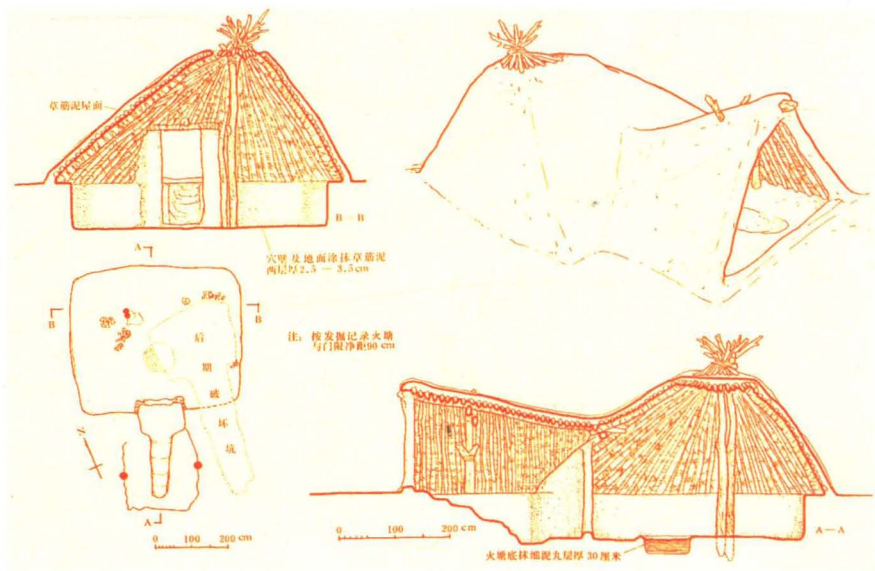
半坡时期的建筑形式
