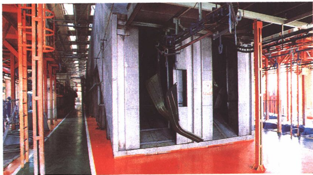
▲双线桥式烘干炉
