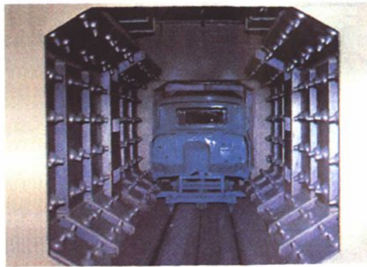
▲面漆强冷室
