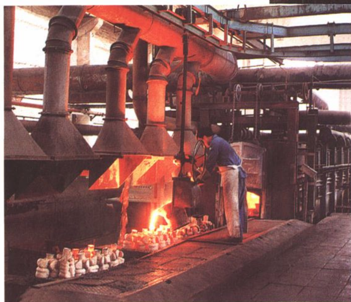
▲精铸模壳焙烧炉
