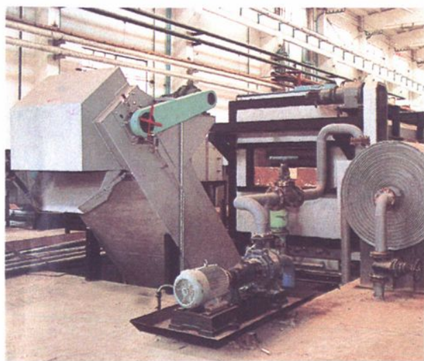
▲ 750kg 级铸链输送带式调质线
