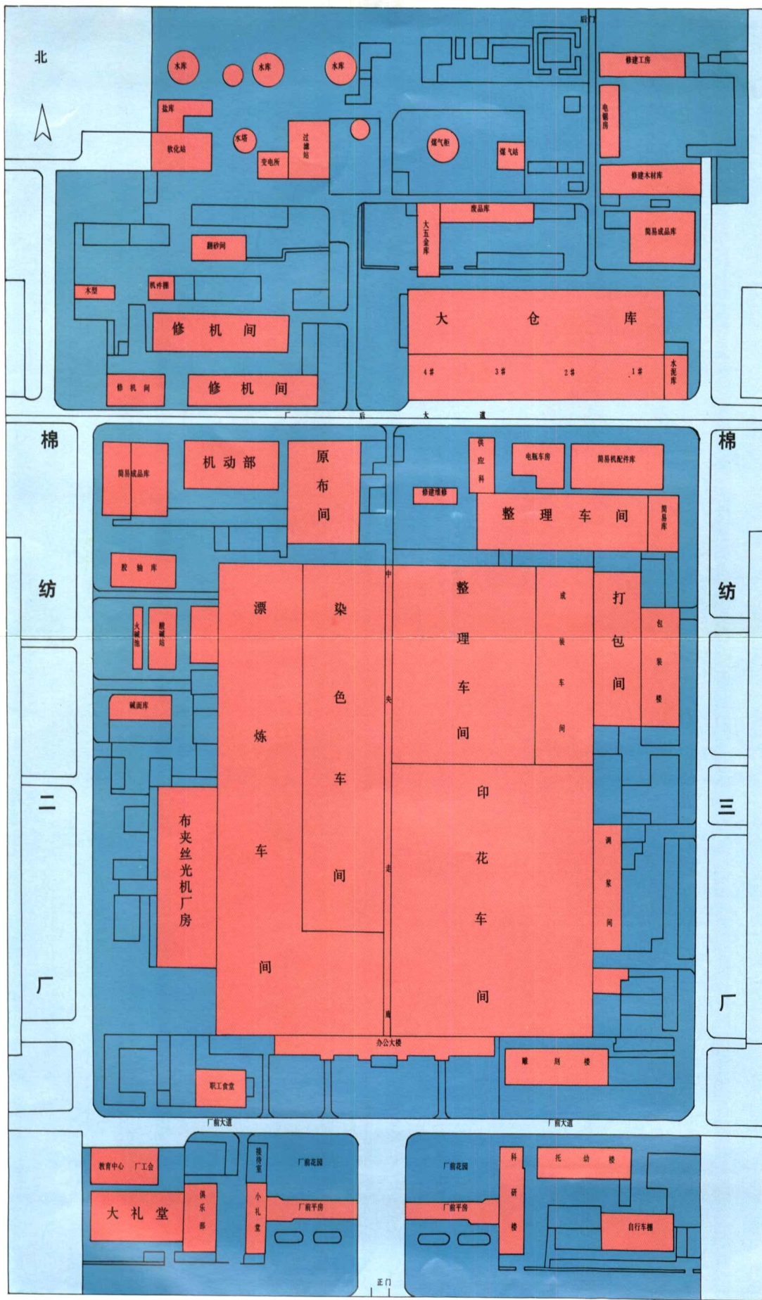
石家庄第一印染厂 厂区平面图
