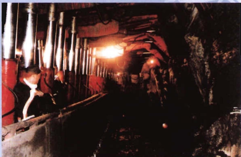
▶ 综采工作面
