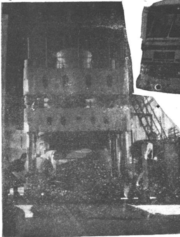
◀ 客车厂首家使用的双动式油压机
