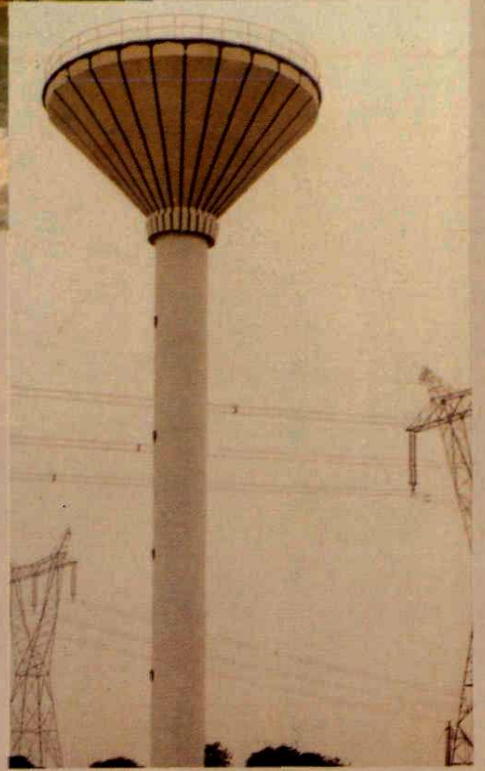
抽取 152.8 米深层地下水， 日产水量 3 千吨的人和自来水厂
