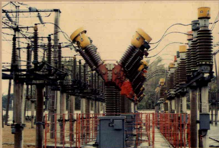
座落在鹤亭的 110 千伏设计容量 8 万千瓦的变电站
