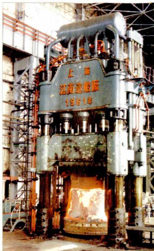
万吨水压机
