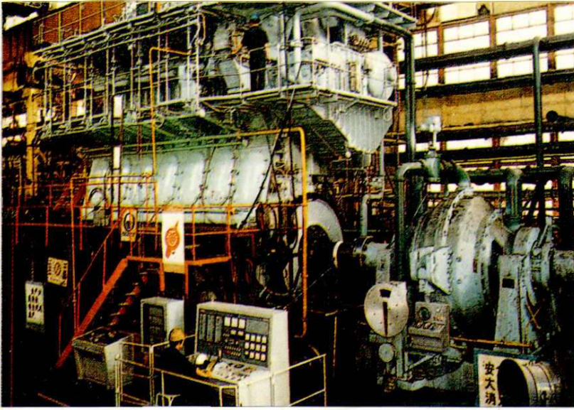
HD-M.A.N/B&W6L60 型柴油机
