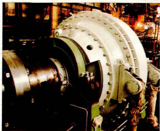
水力测功仪
