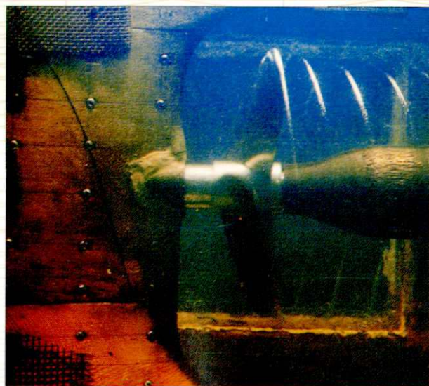
空泡水洞
