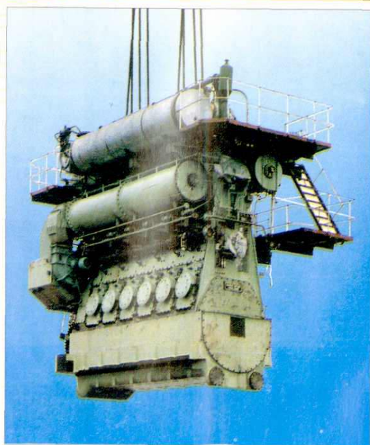
出口巴西 7RTA48 船用低速柴油机
