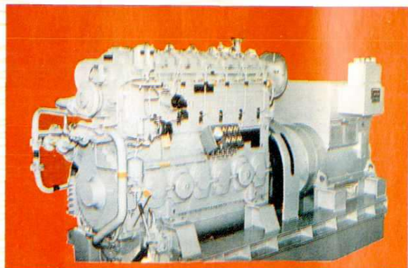
CXZ-M.A.N/B&W20/27 柴油机
