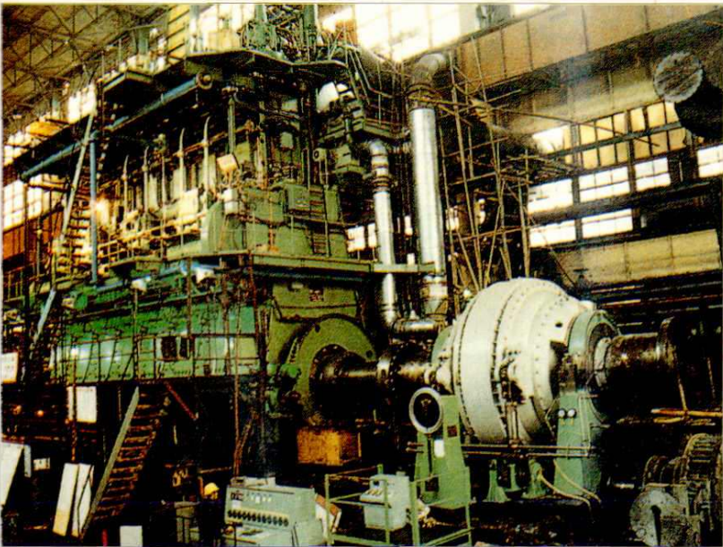
沪东造船厂、上海船厂合作制造苏尔寿7RTA84+EB型船用低速柴油机
