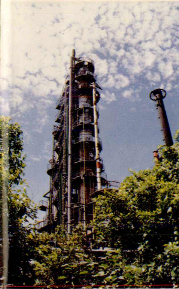
南充炼油厂同轴式催化裂化装置
