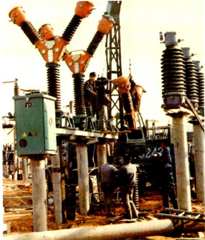
右图 变电工区 工人在北门变电站安 装油断路器
