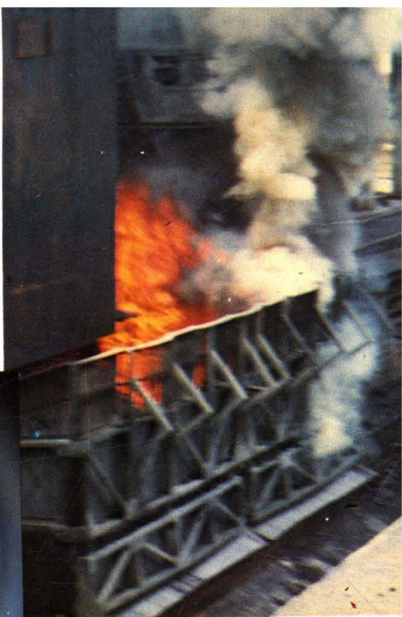
焦化煤气总厂炼焦炉
