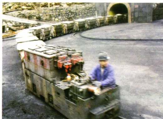
赤水市岔角煤矿一角 (2006年摄) (图51)
