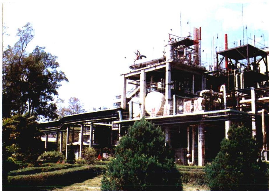
福州第二化工厂聚氯乙炔高型号生产装置
