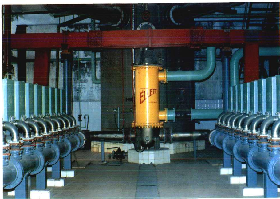
福州第一化工厂引进芬兰诺基亚化学公司1万吨/年氯酸盐电解槽装置
