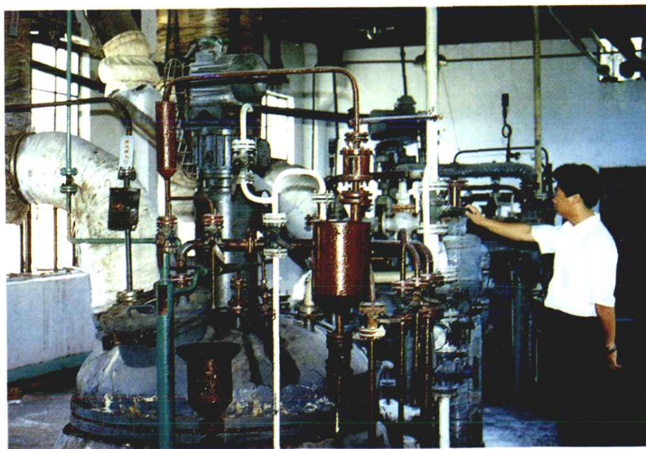
福州医疗化工总公司 5000 吨 / 年增塑剂生产装置
