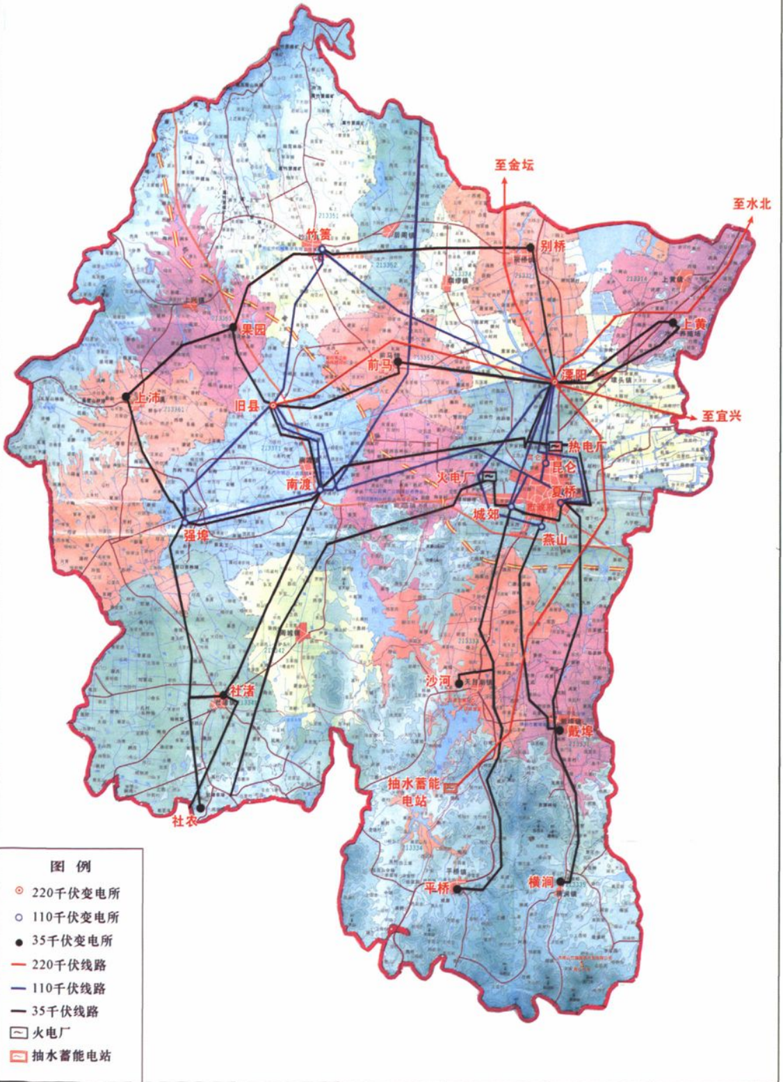
2002年溧阳市35千伏及以上电网地理接线示意图
