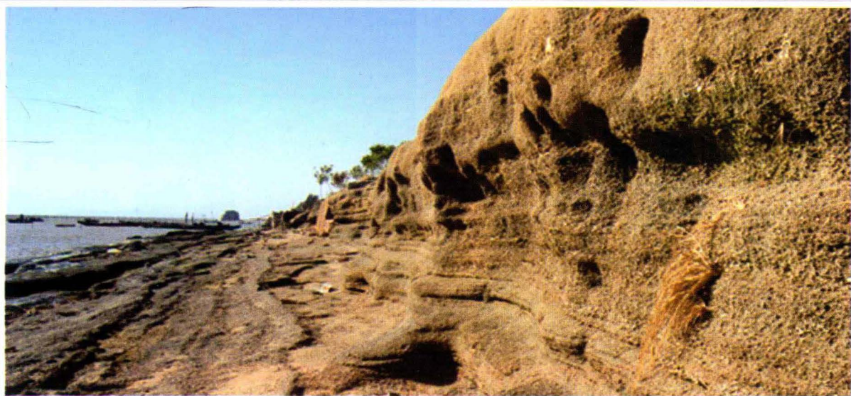
海山岛海滩岩（2010年摄）
