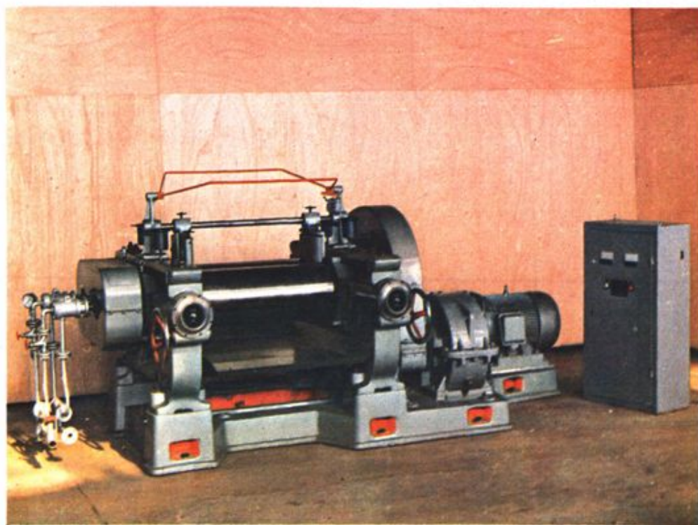
SK-400B开放式炼塑机
