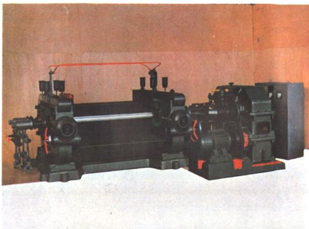
SK-550开放式炼塑机
