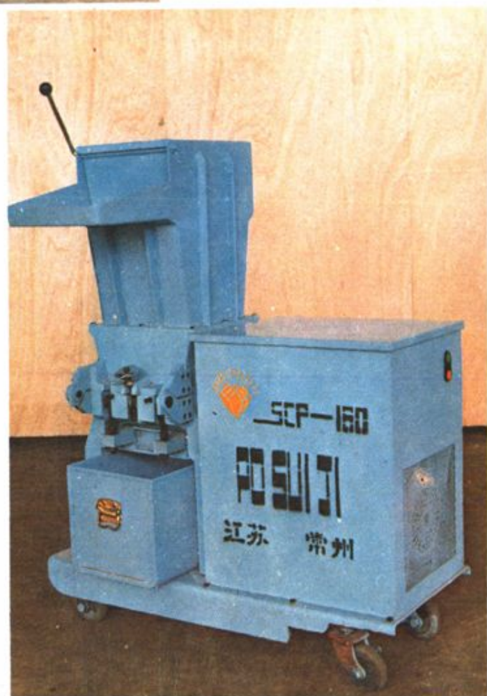
SCP-160·280塑料破碎机
