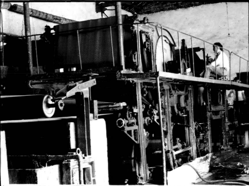
大屏山煤矿瓦楞纸厂造纸机
