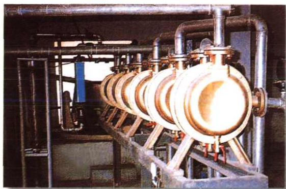
马铃薯淀粉生产线
