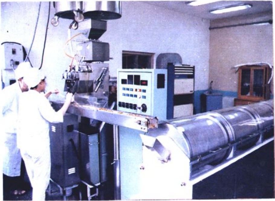
本设备是八五年从意大利进口软胶丸装封机全自动
