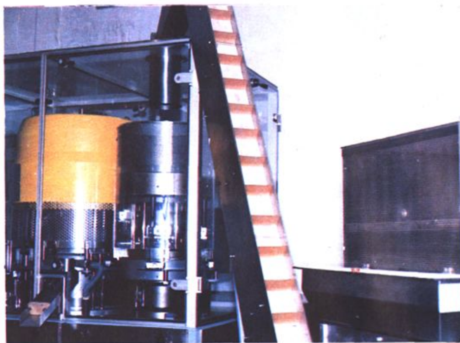
本设备是从意大利进口硬胶丸灌装机
