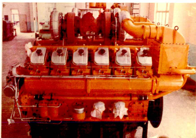
▶ 190 柴油机
