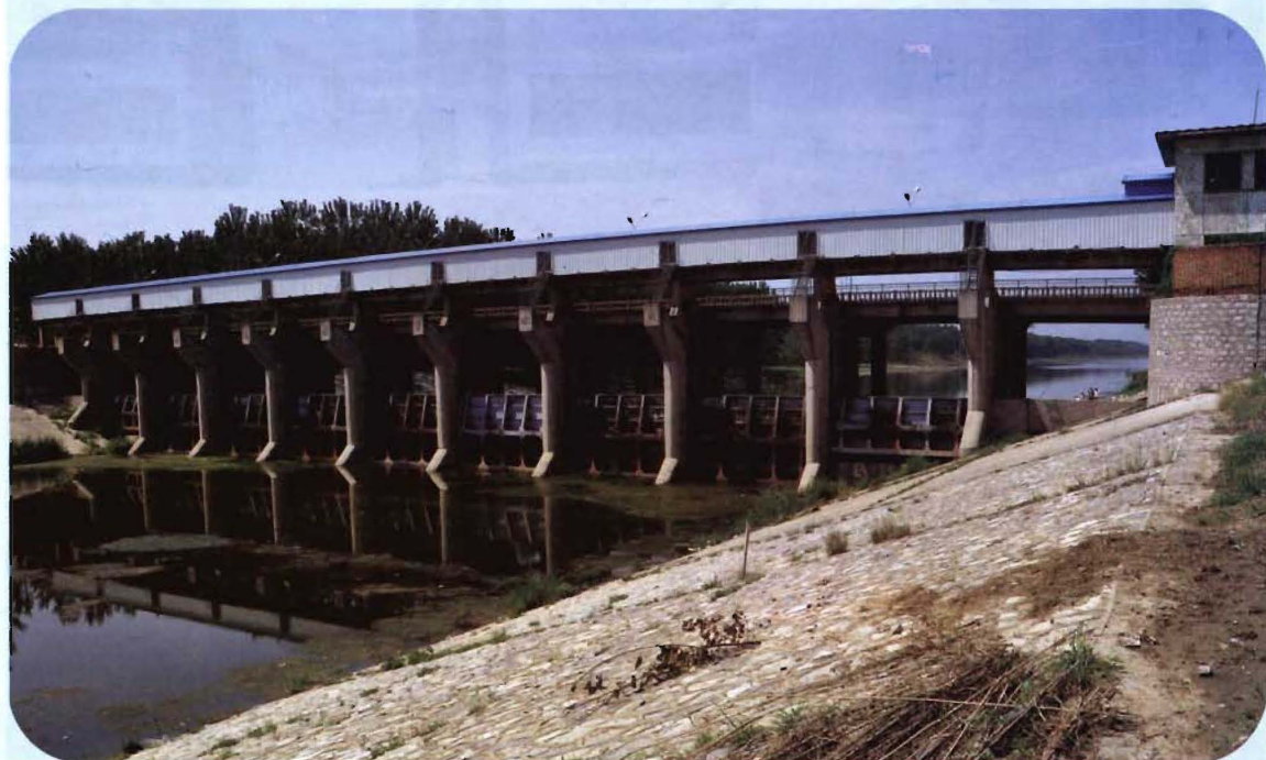
西码头蓄水闸（拍摄于2011年9月）
