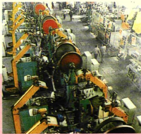
湖北气门厂的自动气门毛坯生产线
