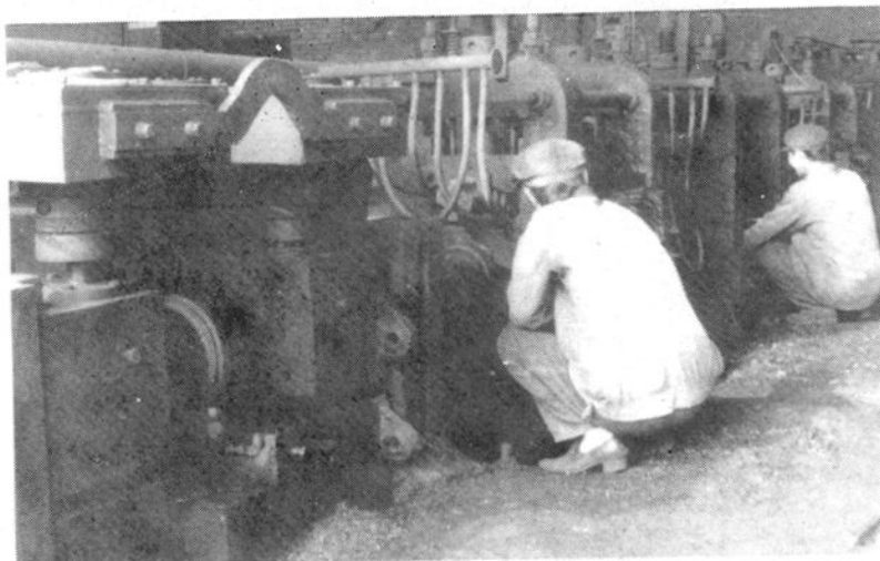
型钢厂自行设计安装的GY-3型短应力线轧机，1985年获省重大科学技术研究成果三等奖。图为工人在维修机器。
