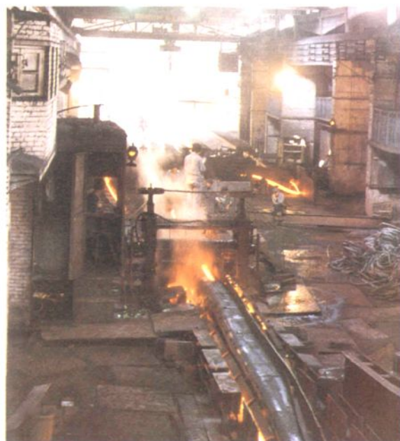
400/250 机组生产场景
