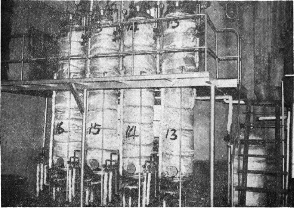
无水酒精生产设备——脱水干燥塔
