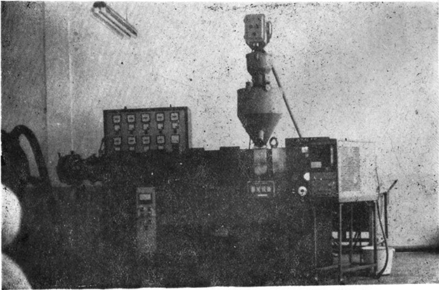
从意大利引进的PVC薄膜成套专用设备（局部）
