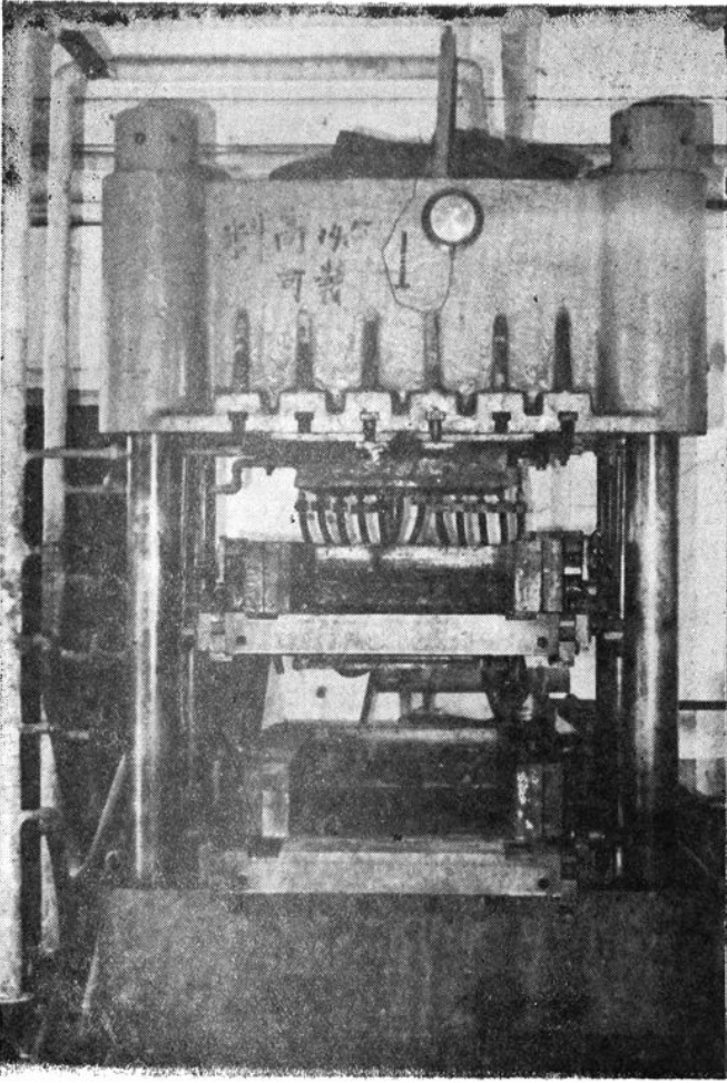
赛片生产设备 —压块机
