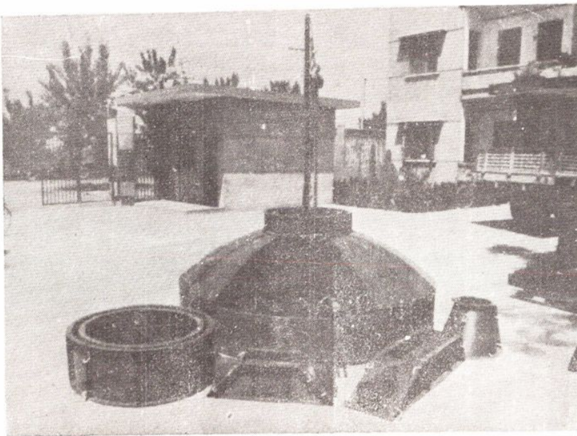
混凝土沼气池钢滑模
