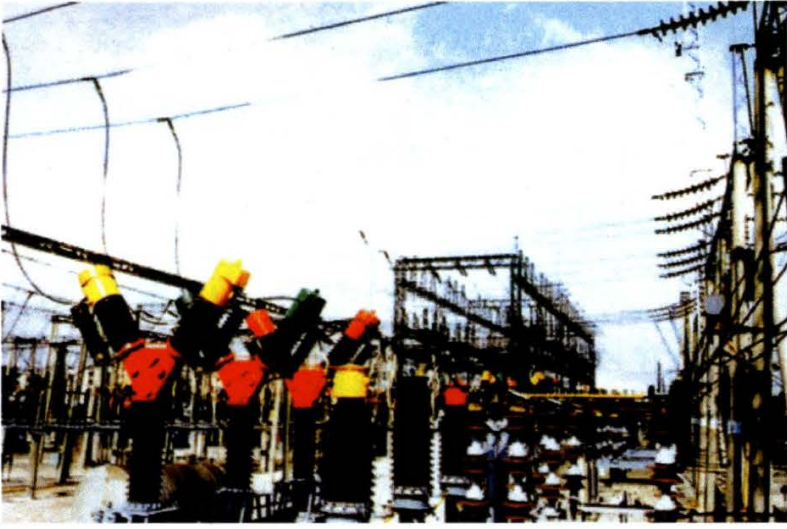
1967年投运的江苏省首座220千伏变电所——常州变电所
