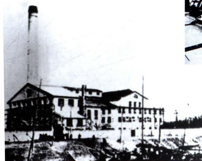
1933年戚墅堰电厂发电所主厂房
