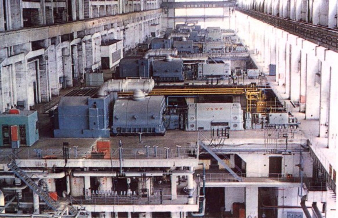
发电机组
