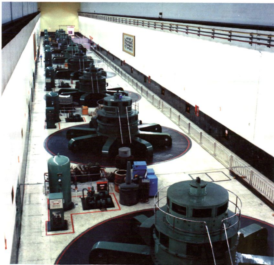
发电厂房
