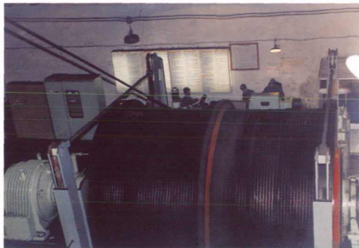
锡铁山二矿育井 \phi 3.5\text{m} 竖井卷扬机
