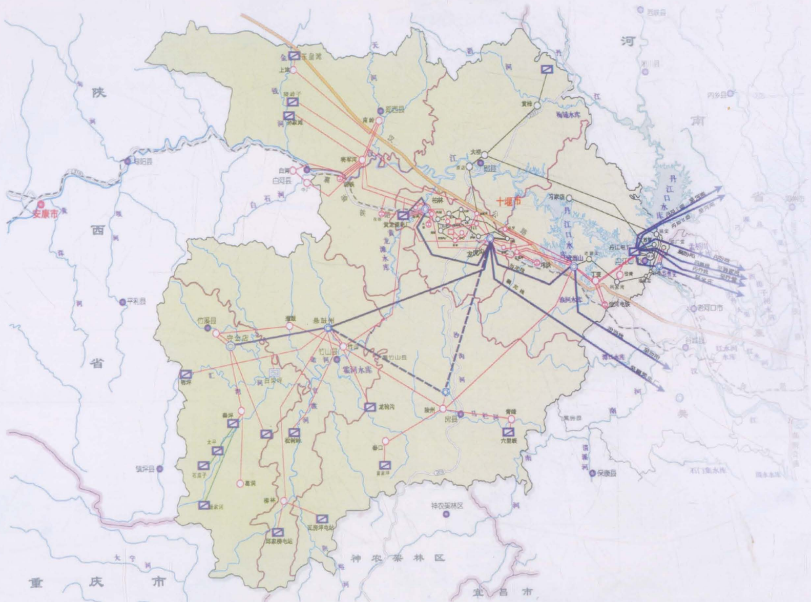
十堰电网2008年地理接线图
