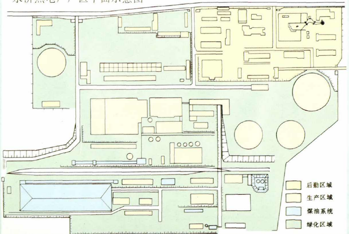
永济热电厂厂区平面示意图
