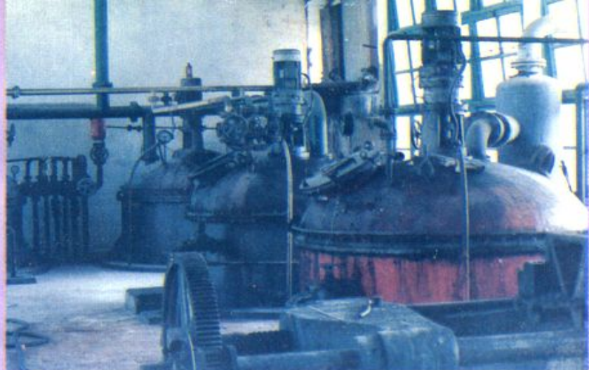
◀ 市西合粮库肌醇 生产车间
