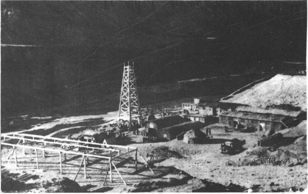
从延长来玉门的顿钻正在钻第一井
