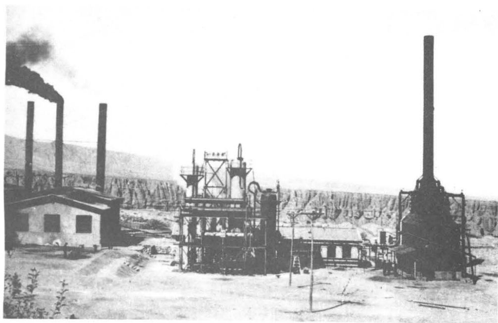
1947年在四台建成的裂炼装置
