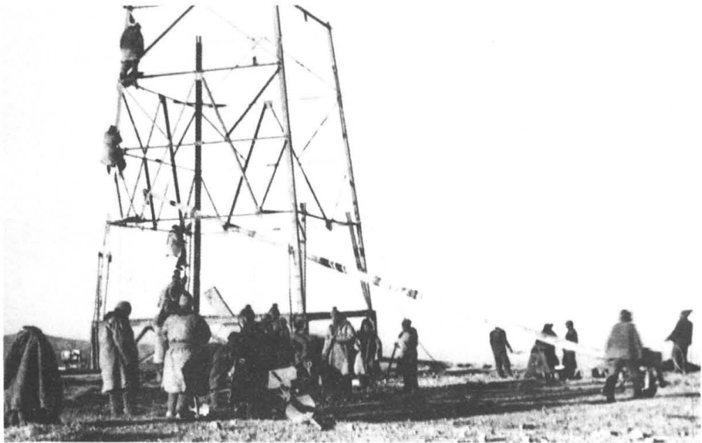
工人们冒着严寒安装井架
