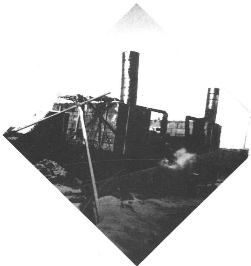
安装于12井选油站的木制油气分离器
