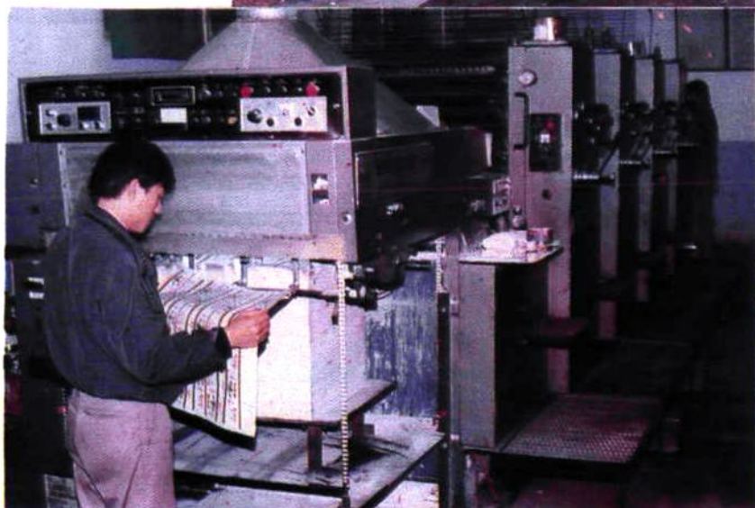
四色对开胶印机 PZ4880-01A
