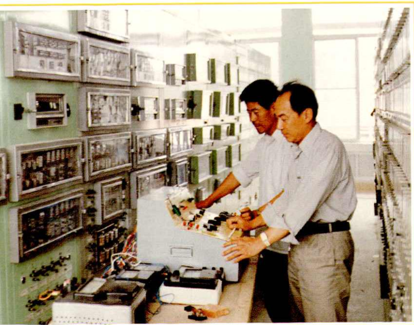
进行继电保护试验
