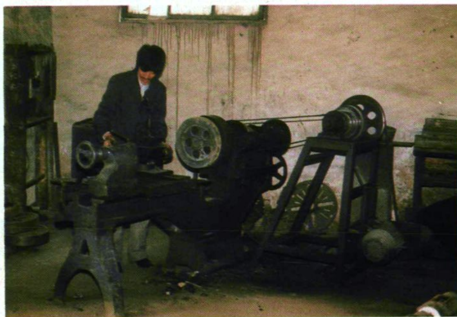
这台旧皮带车床是皮革机械厂老技工冯贵五十年代初从天津购回的它是曲沃手工业机械化的开端
