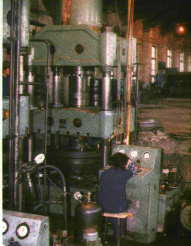
300吨油压拉伸机压制“钢瓶”外壳
