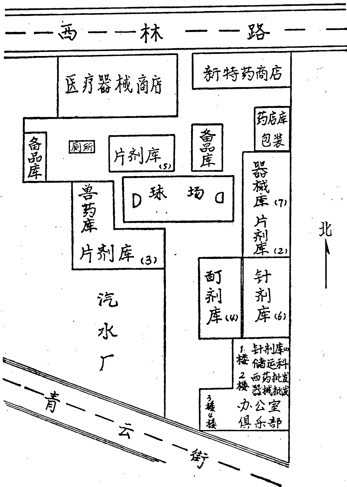
佳木斯市医药公司平面图
