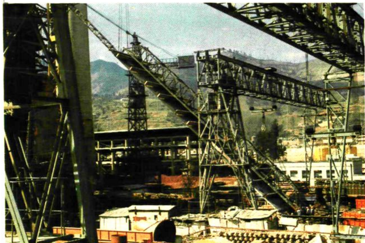
410吨/时锅炉水冷壁吊装
