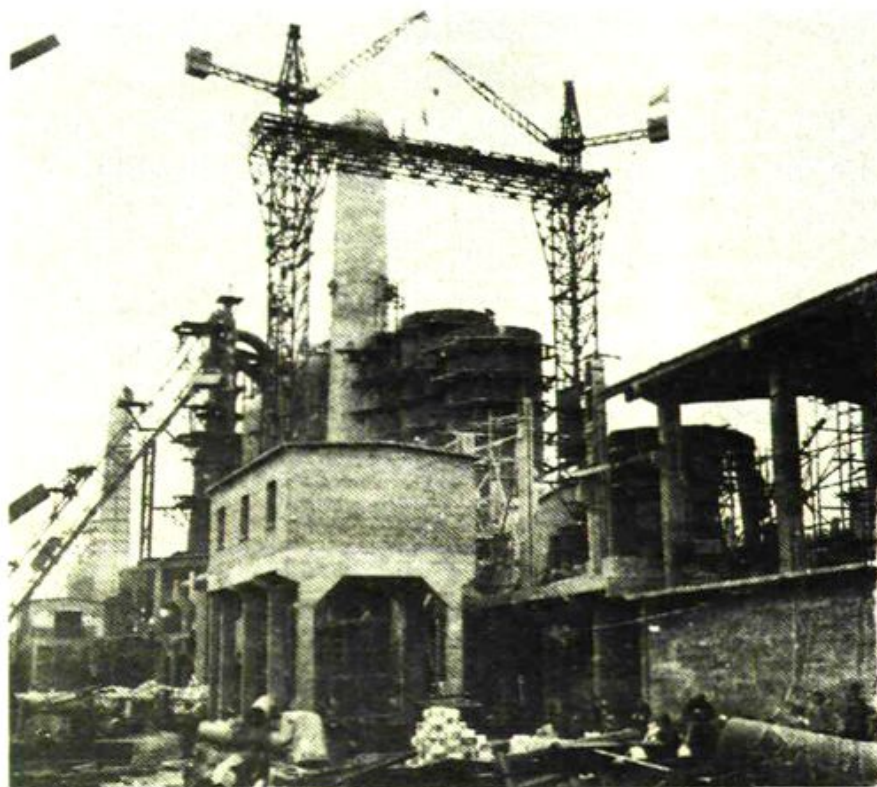
昆明钢材公司扩建2号高炉、自制的龙门塔式吊车
