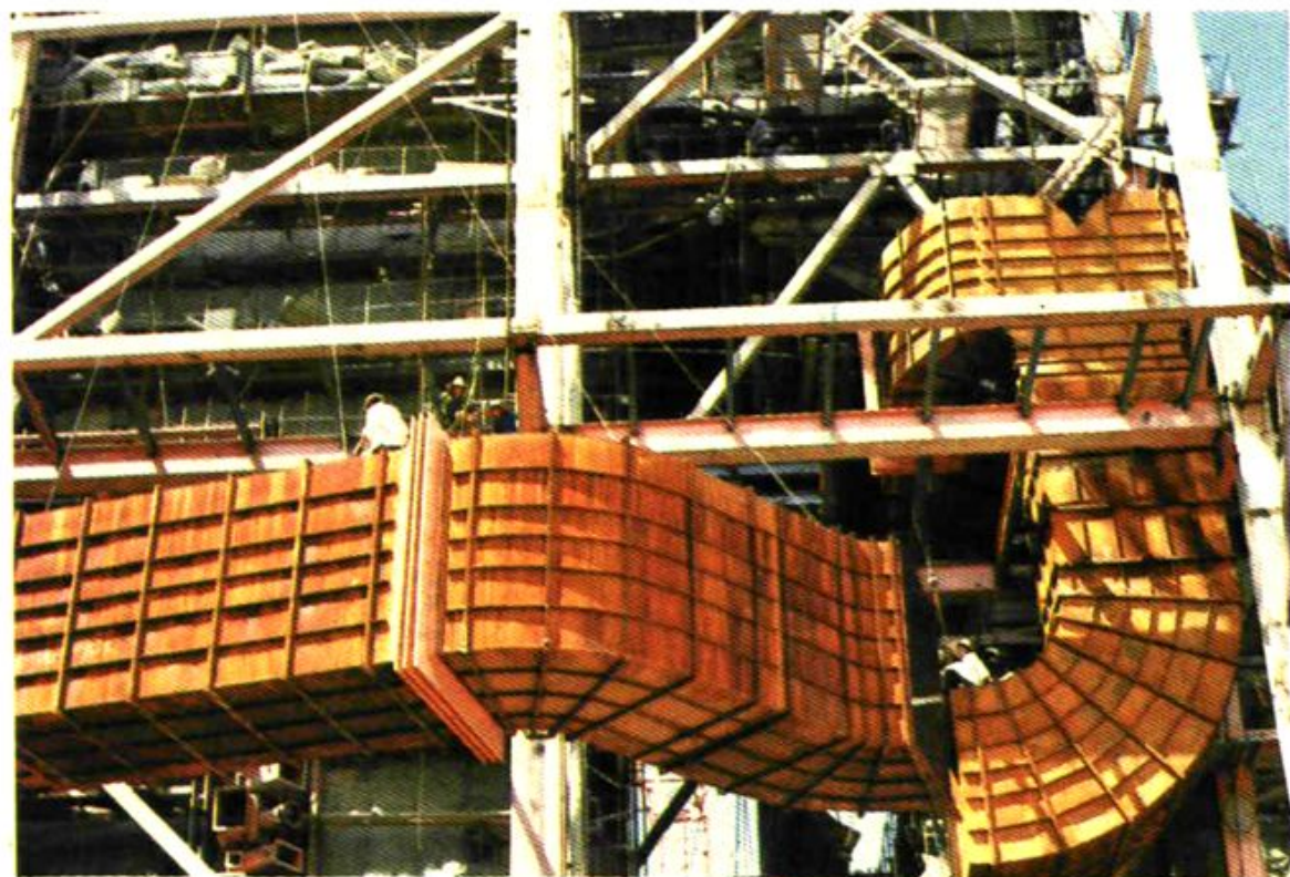
410吨/时安装通风管道
