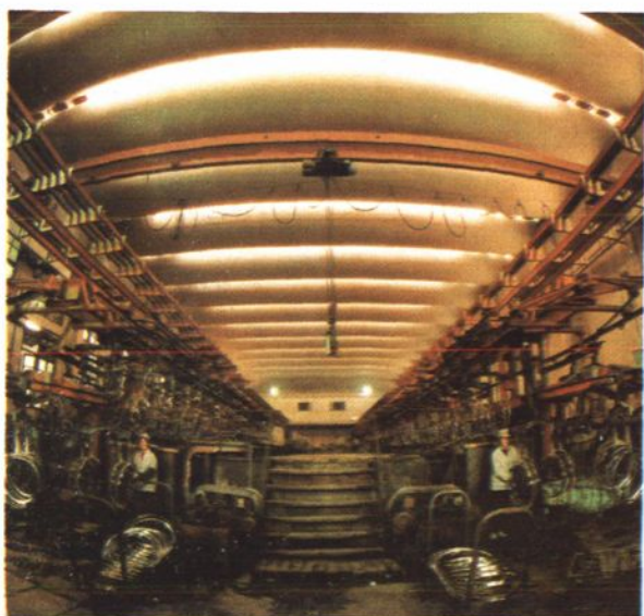
电镀环形生产线
