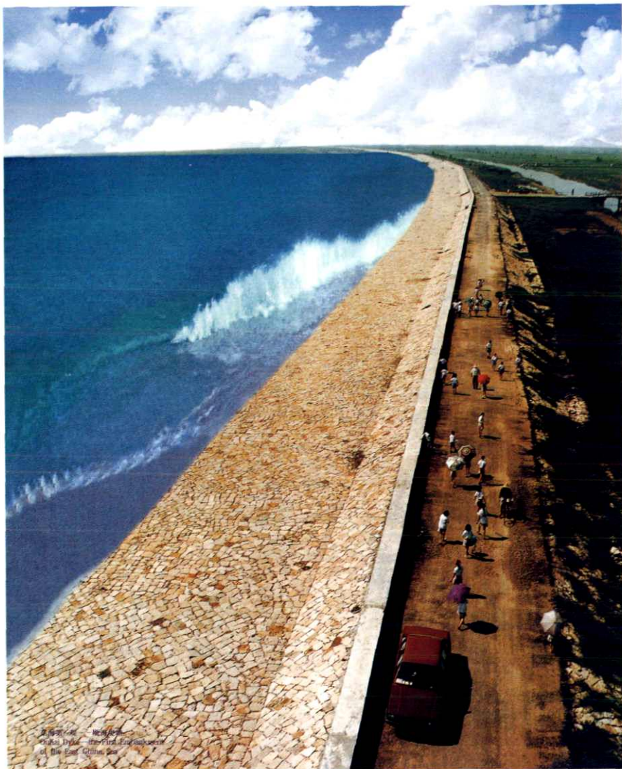
瓯海区永强标准海堤
