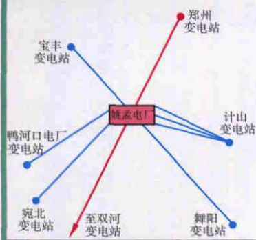
姚孟电厂与电网接线示意图
