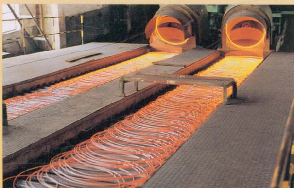
石特钢厂线材（直条）生产线
