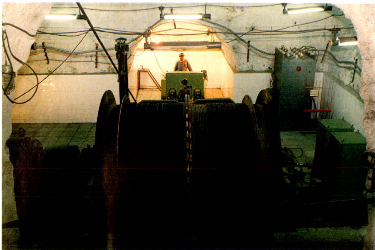
井下提升机机房
