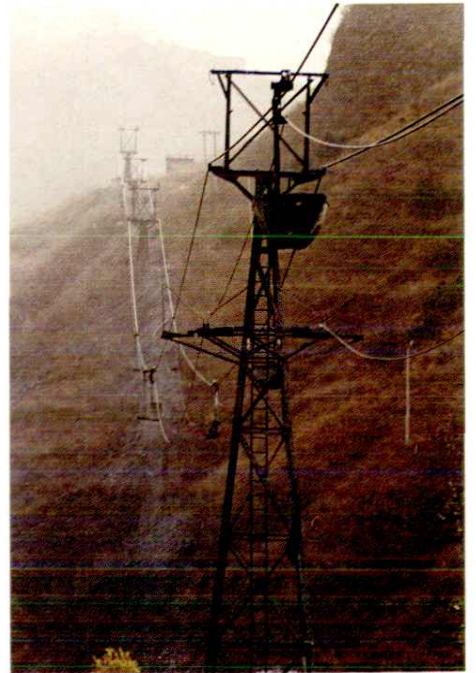
房山矿高架索道排矸
