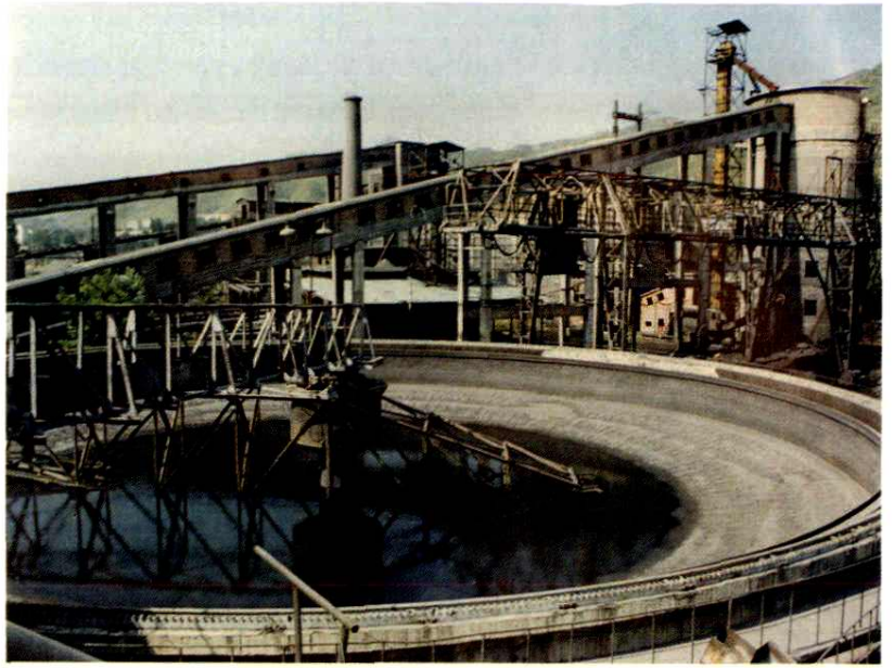
房山矿水采煤沉淀池
