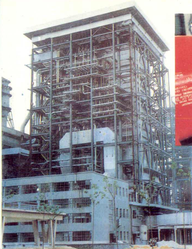
△东方锅炉厂生产的配 30 万千瓦机组亚临界自然循环汽包锅炉在山东邹县电厂投产
