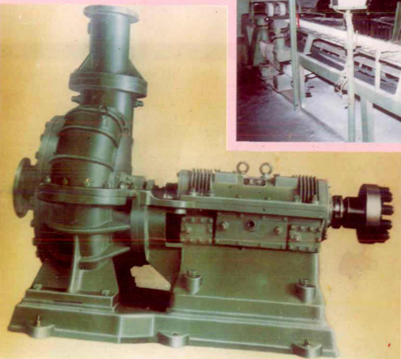
△自贡工业泵厂荣获机电 部科技成果三等奖的 10PH(GS)二级串联 灰渣泵
