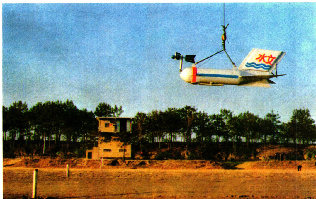
洙赵新河梁山闸水文测流
