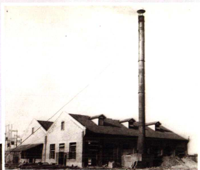
民国 8 年（1919 年），嘉兴永明电气股份有限公司建造的发电车间和 120 千瓦卧式蒸汽发电机组
