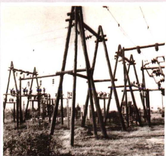
1957年7月28日投运的35千伏长安变电所
