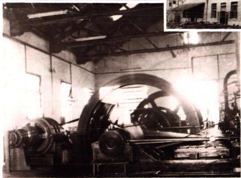
民国 8 年（1919 年），嘉兴永明电气股份有限公司建造的发电车间和 120 千瓦卧式蒸汽发电机组
