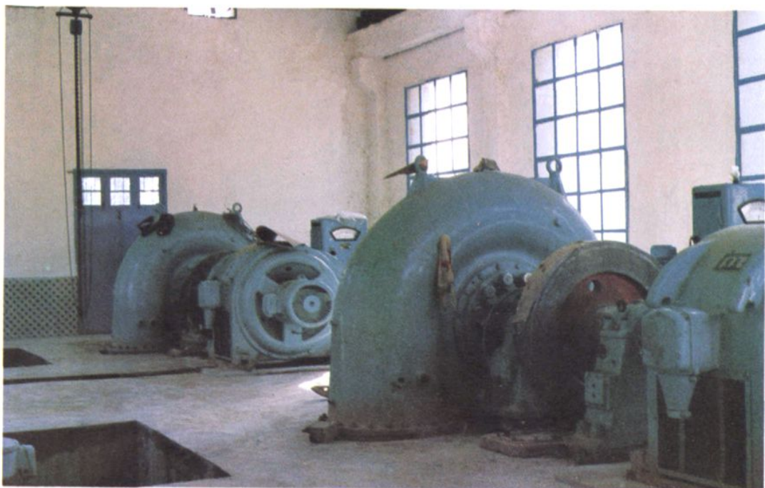
人行元阳县支行贷款建设的元阳县黄金工业公司二级电站机组
