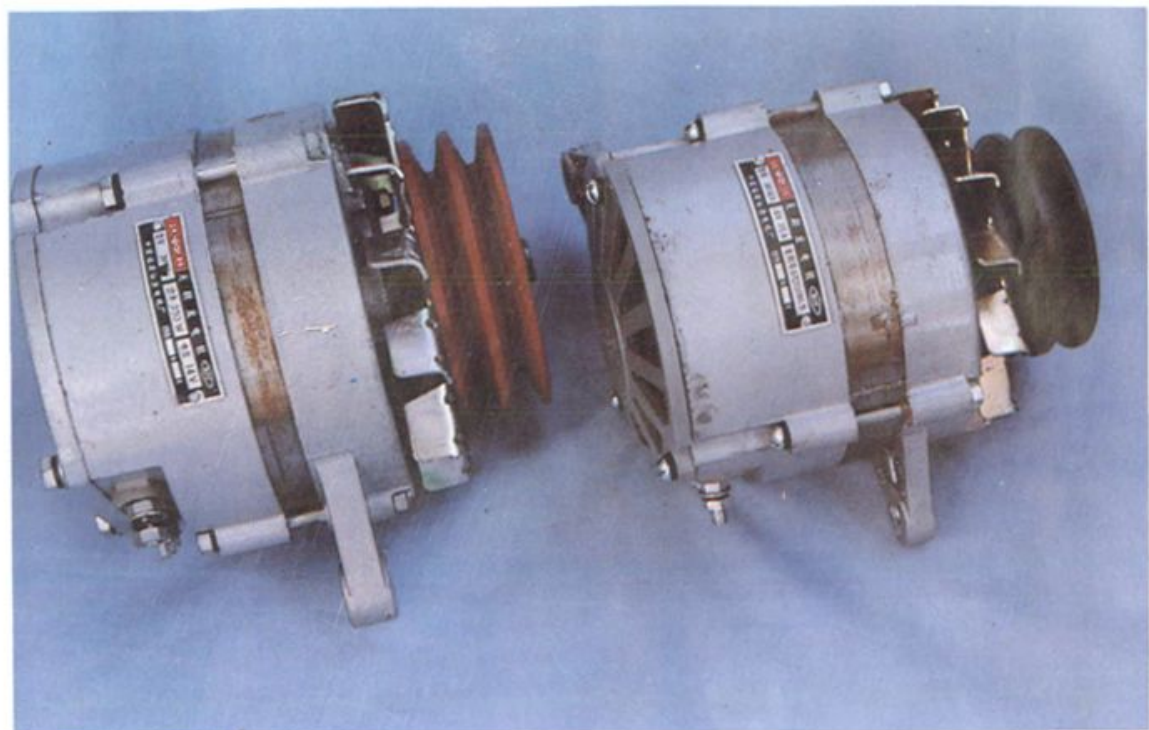
仙游电机厂生产的无刷电机
