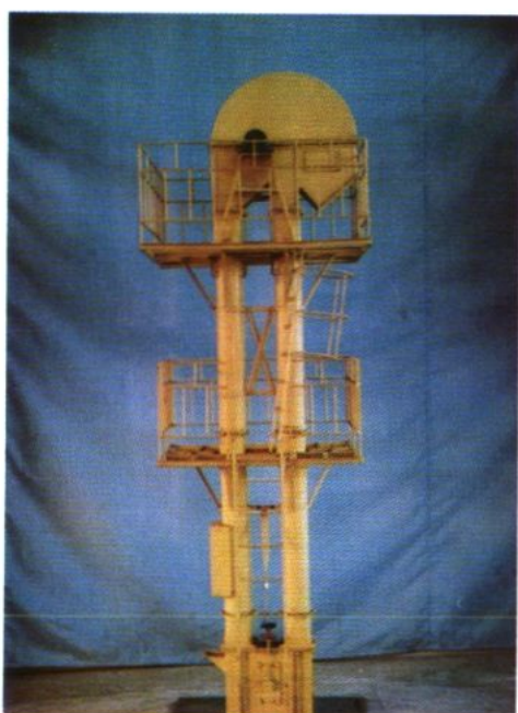
金山粮机厂生产的园型斗式提升机
